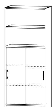
Flexeo® Schiebetüren-Schrank, 5 Ordnerhöhen mit 3 geschlossenen & 2 offenen Fächern Maße (H x B x T): 190 x 80 x 40 cm
